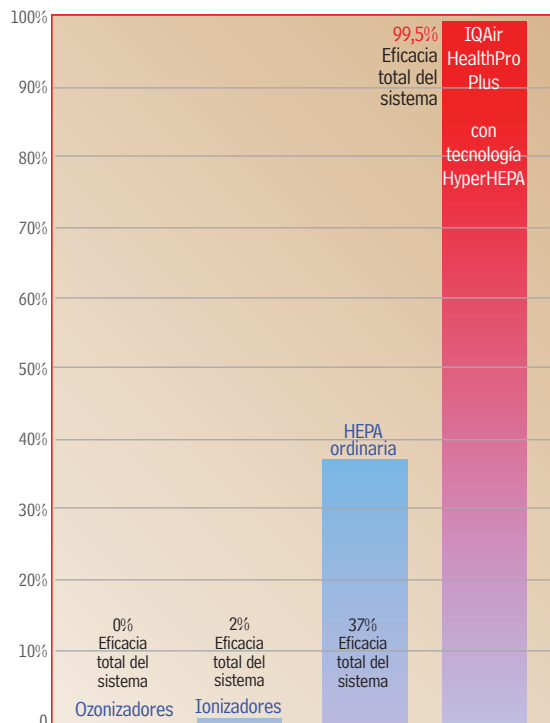
Eficacia total del sistema (retención de partículas) para tamaños de partícula: 0,01 – 1,00 micrones
